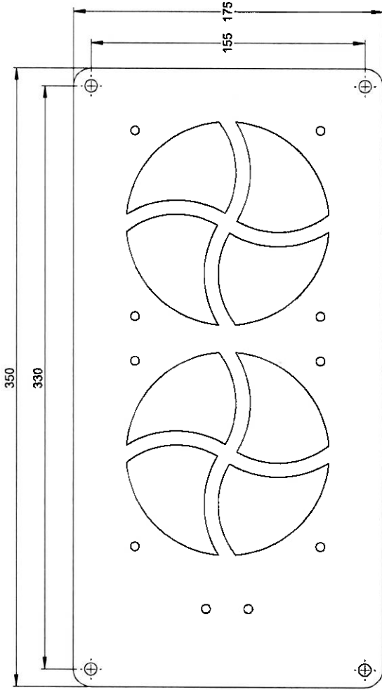
FLAT PATTERN PROFILE # PKTwin Fan Plate-0
